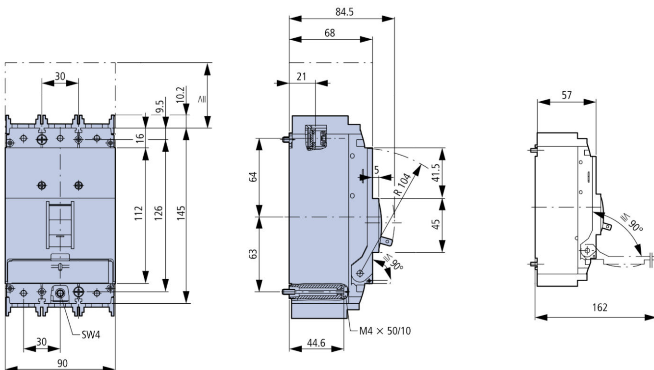
Чертеж: Прекъсвач с лят корпус Тип М, 3Р, 100kA, 40А
