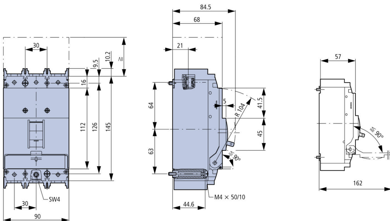
Чертеж: Автоматичен прекъсвач MC1 Тип M, 3P, 50kA, 63A
