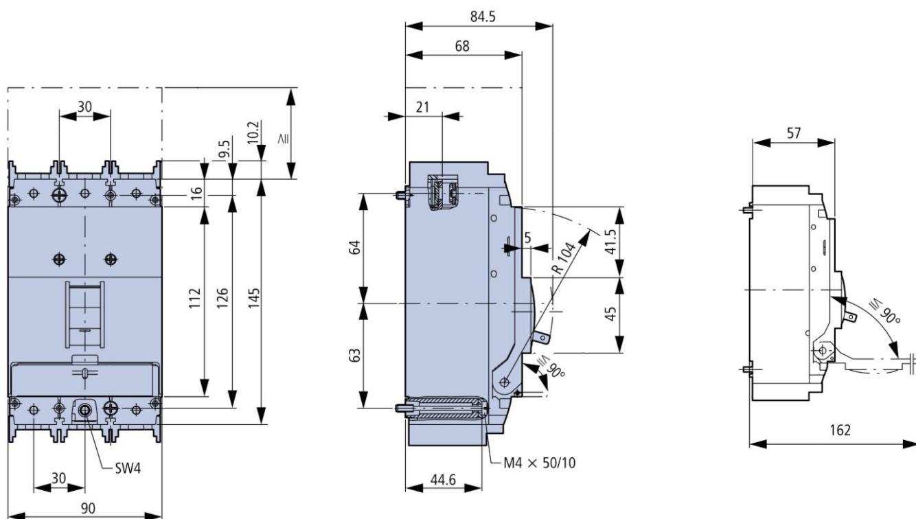
Чертеж: Прекъсвач с лят корпус Тип М, 3Р, 100kA, 63A
