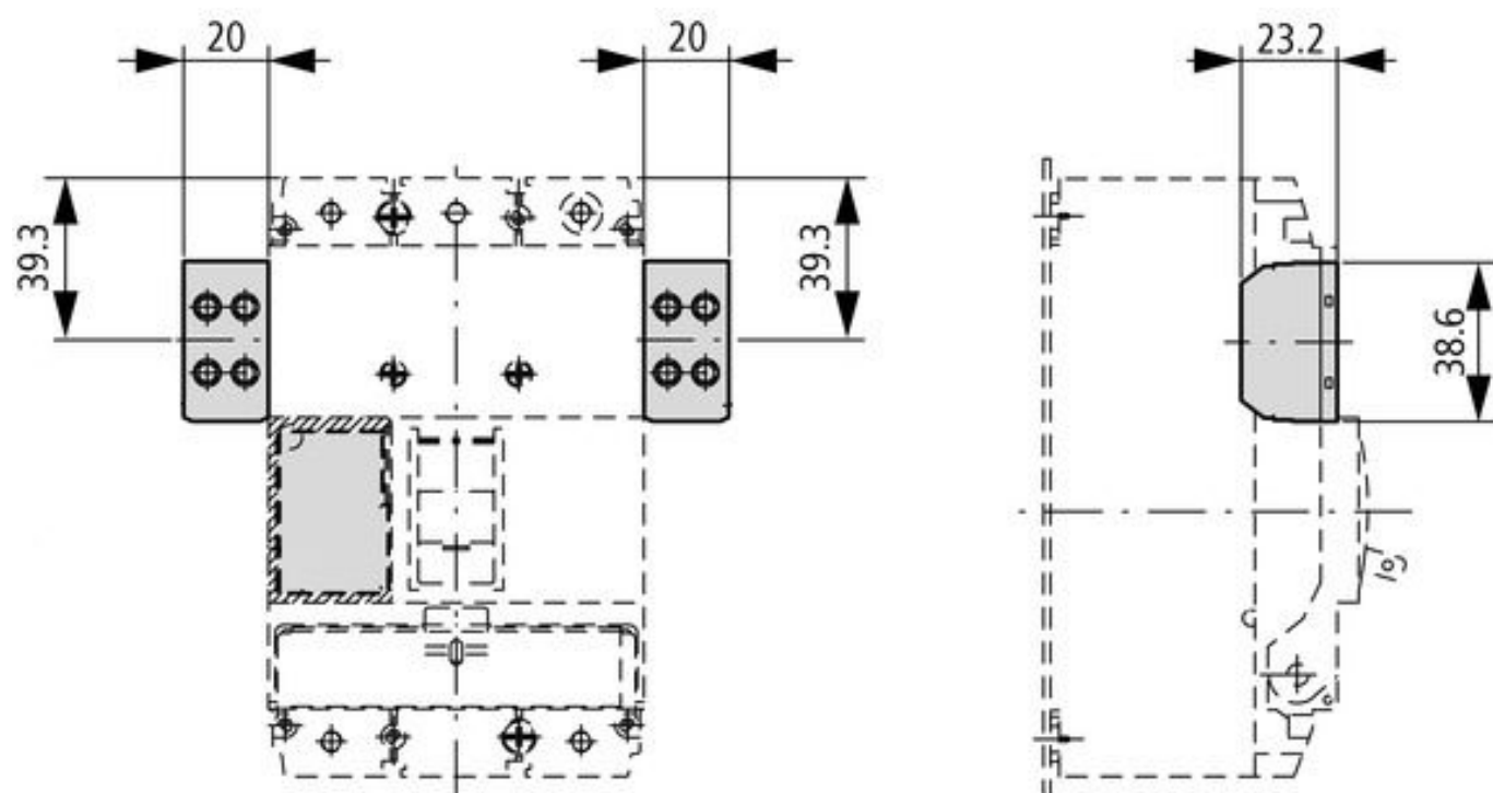
Чертеж: Минимално U изключвател за времезакъснително реле, MC1
