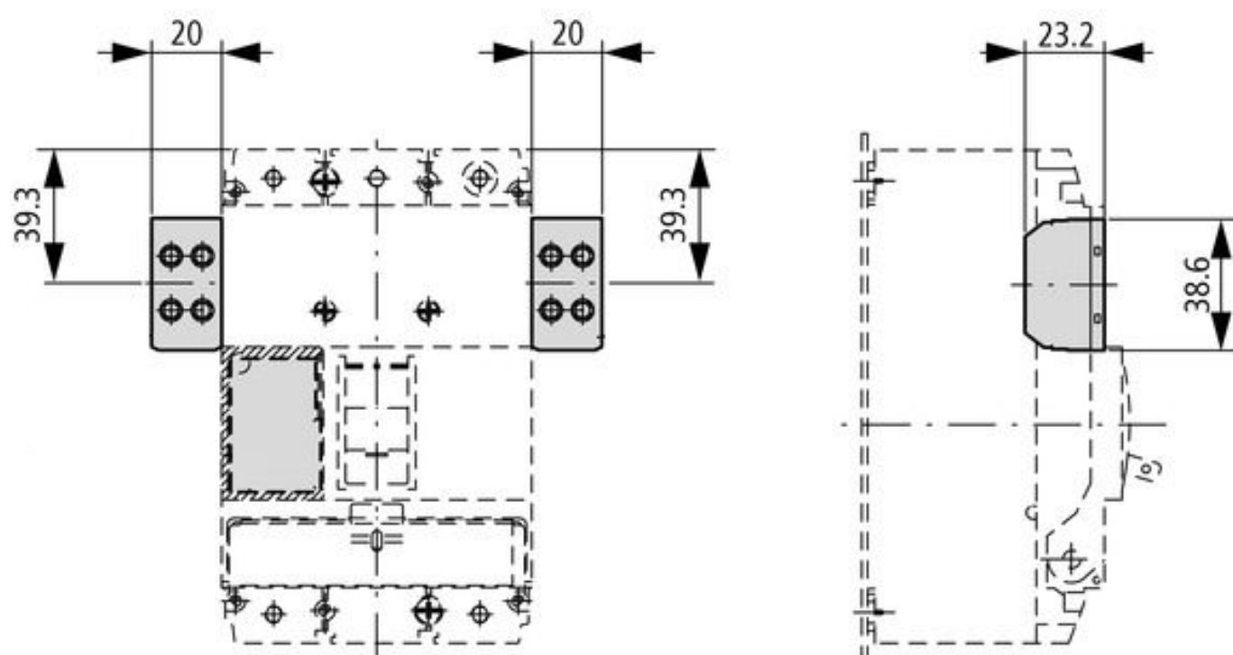
Чертеж: Мин.напрежен ов изключвател 220-250VDC за MC1, с 3m кабел
